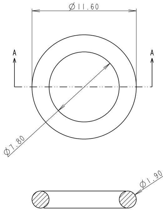
剖面 A-A
