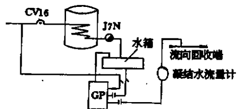
图7 从加热罐中回收凝结水 (行业对象:电力、石油精炼和化学等)
