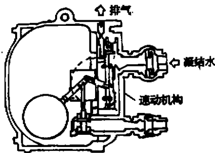
图5 速动机构
