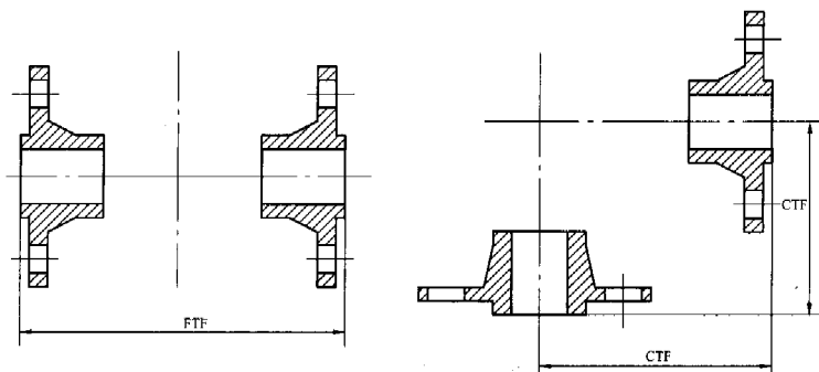
图 1 端面距和中心至端面的间距
