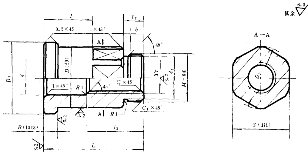
不带滚动轴承的阀杆螺母
