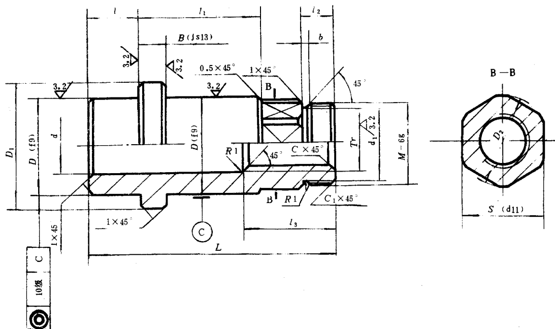
带滚动轴承的阀杆螺母
