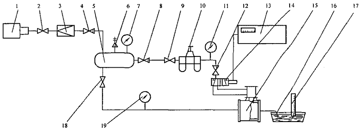
1—空压站(空压机); 2、9、12、18—截止阀; 3—过滤器; 4、8—止回阀; 5—贮气筒; 6—安全阀; 7、11、19—压力表; 10—气源处理装置; 13—切换器; 14—电磁阀; 15—切换阀; 16—水槽; 17—玻璃量筒
