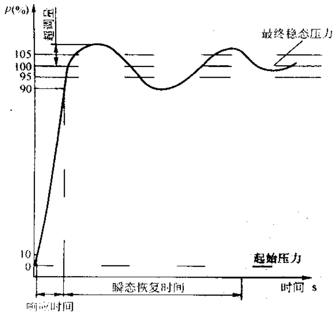
图 A.7 瞬态响应特性曲线
