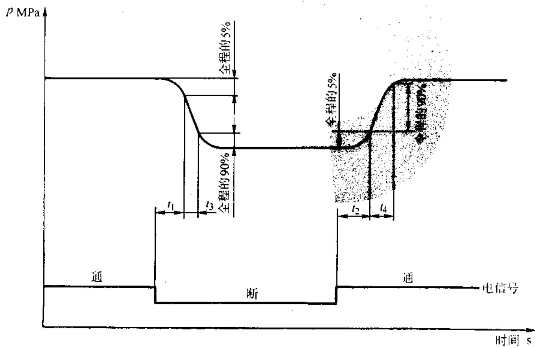
b) 阀芯压力—时间关系曲线
