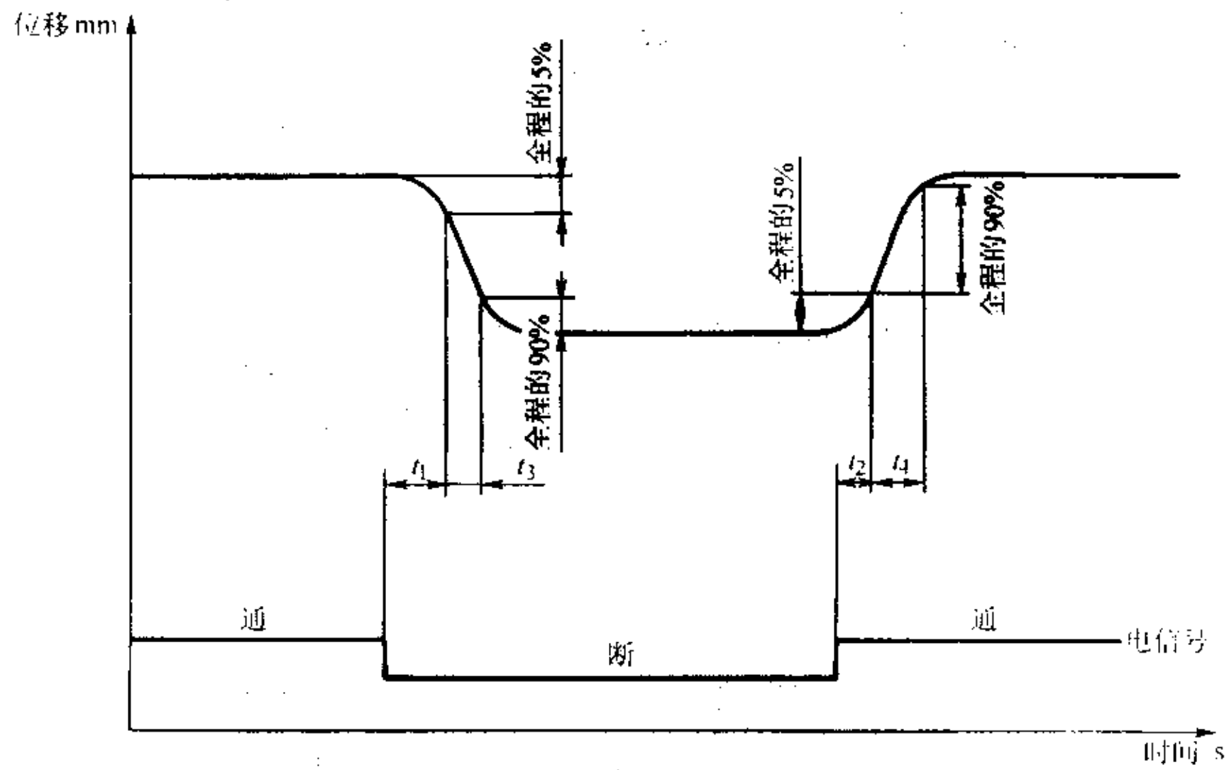
a) 阀芯位移—时间关系曲线
