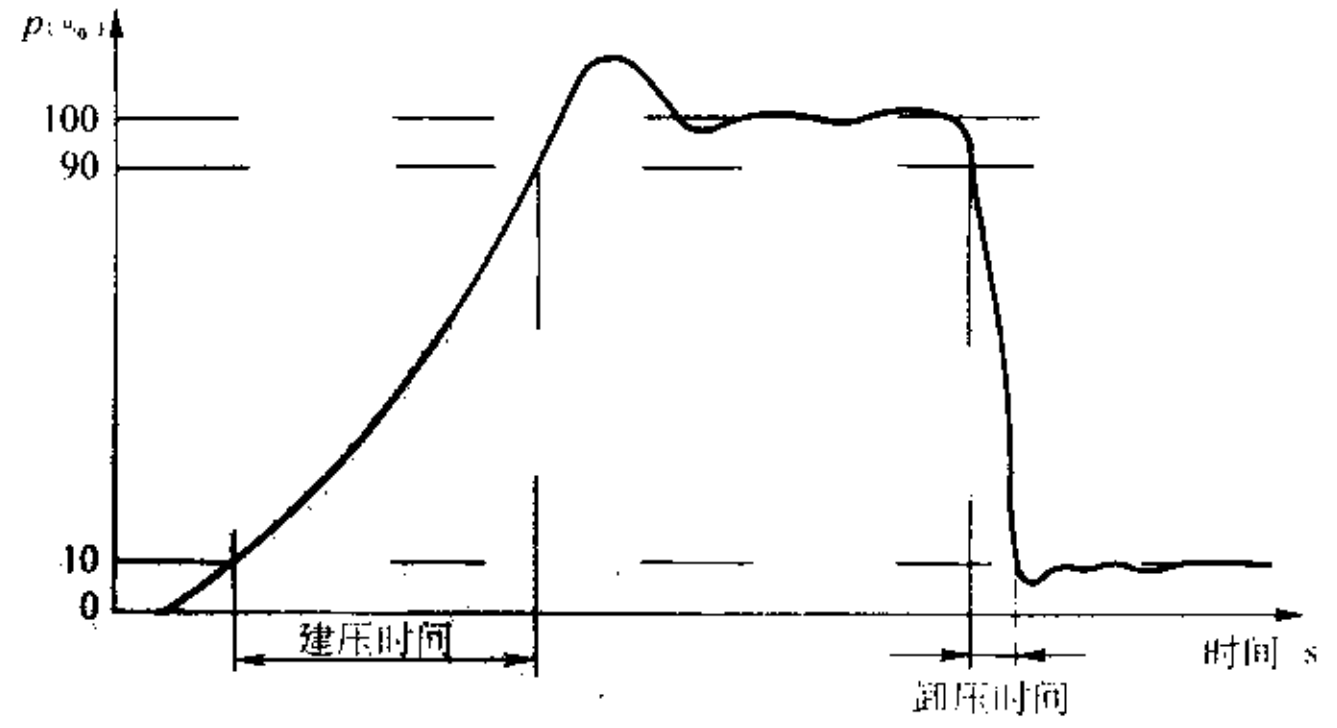
图 A.8 建压、卸压特性曲线
